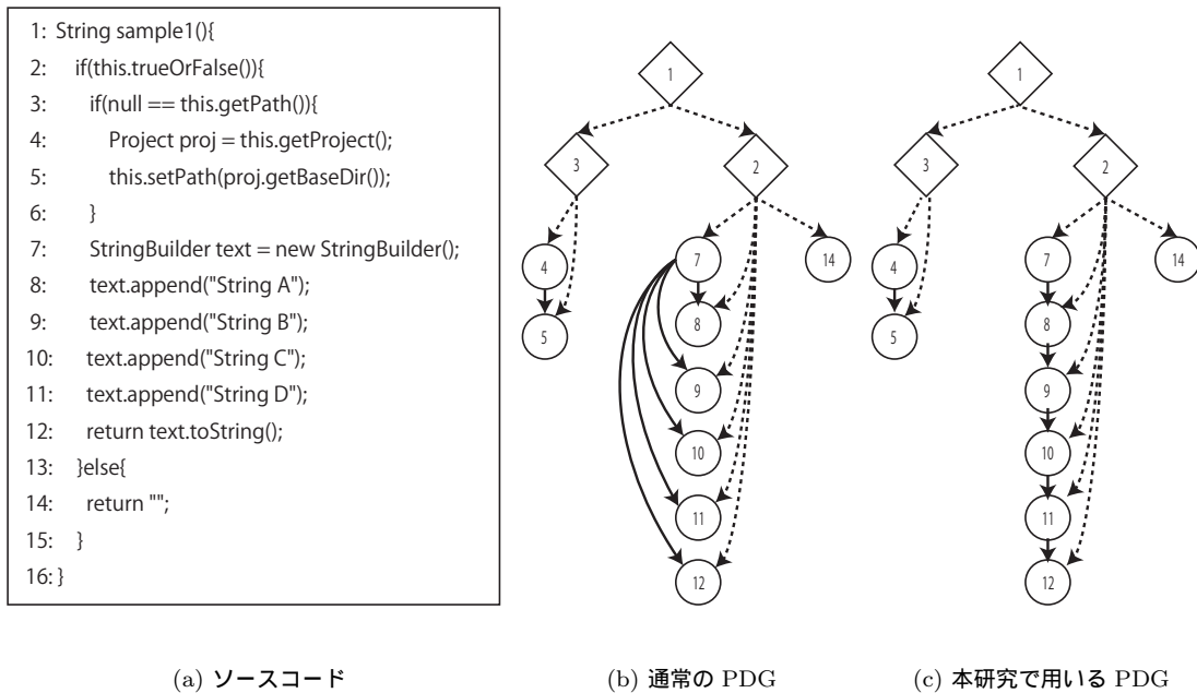
図 1: ソースコードと PDG の例
