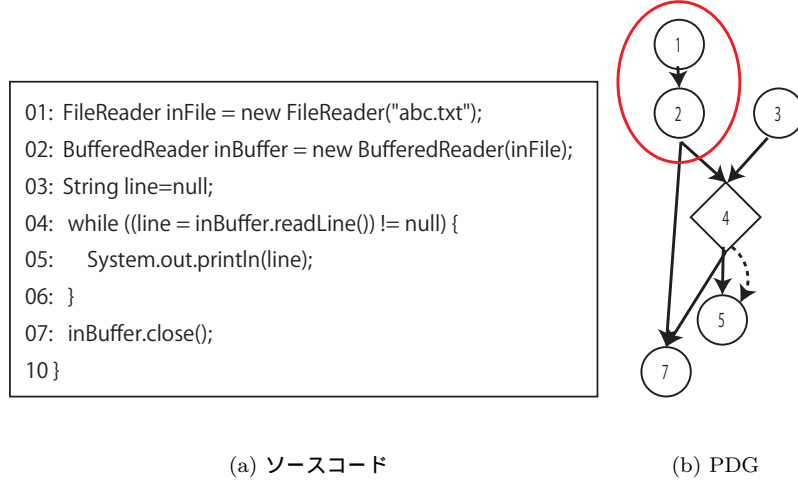
図 4: 提案手法による PDG の配置 (Atomic Data Dependency)
