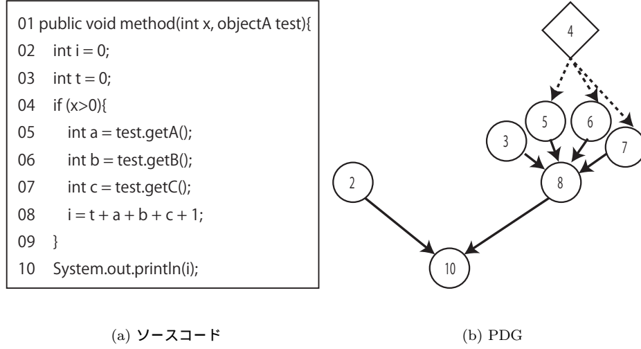
図 3: 提案手法による PDG の配置
