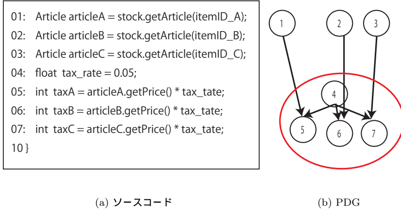
図 5: 提案手法による PDG の配置 (Spread Data Dependency)
