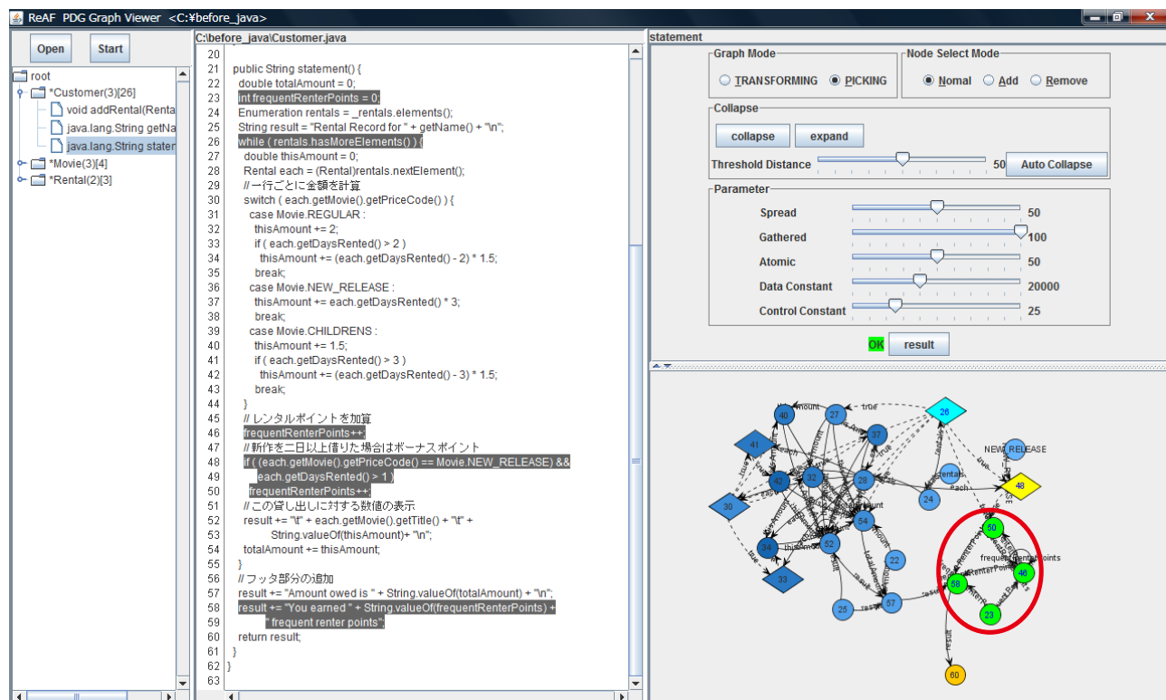
図 7: ReAF のスナップショット
