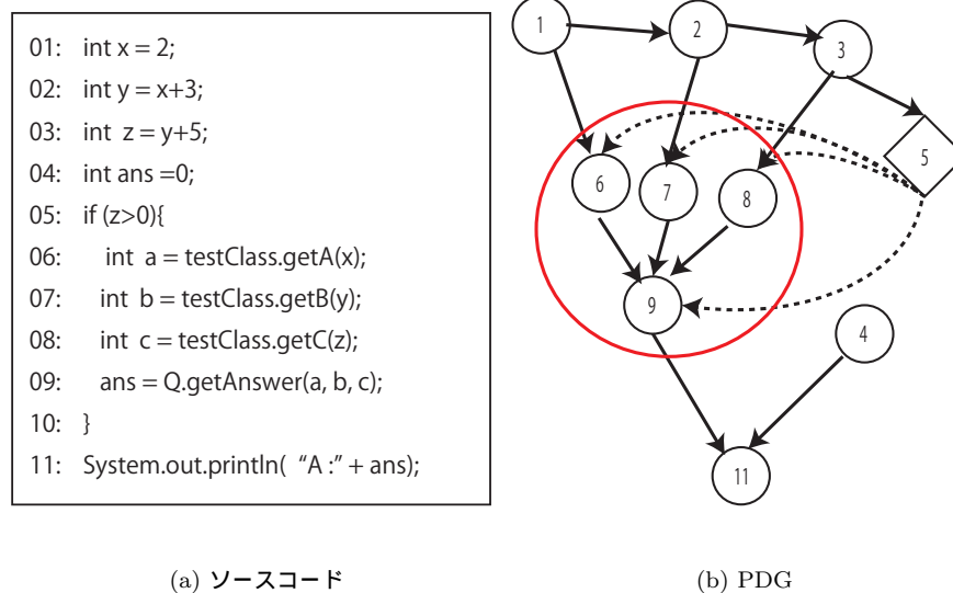
図 6: 提案手法による PDG の配置 (Gathered Data Dependency)
