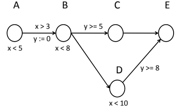
図 5 元モデルの時間オートマトン
