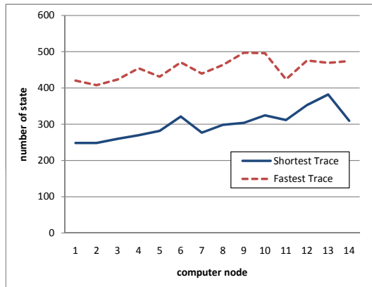
図 10 状態数
