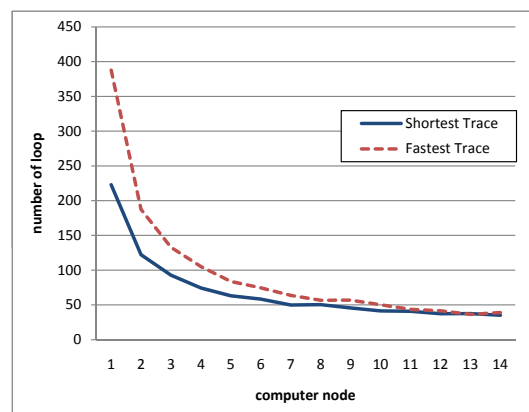
図 8 ループ回数
