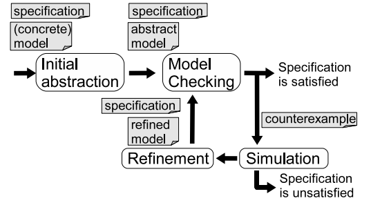
図 1 一般的な CEGAR アルゴリズム
