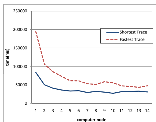
図 9 処理時間
