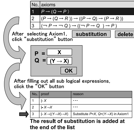
図 3 代入の流れ
