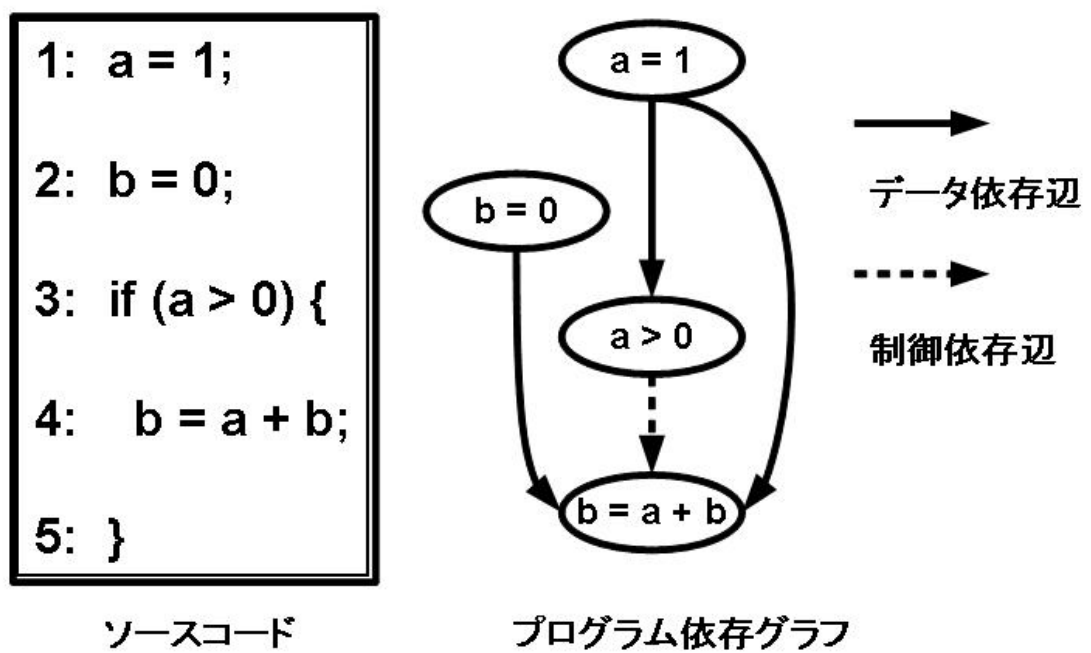
図 1: プログラム依存グラフ
