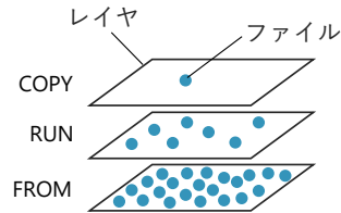
(b) 構築される Docker イメージ
