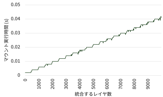
図 3: 統合するレイヤ数と OverlayFS マウント実行時間
