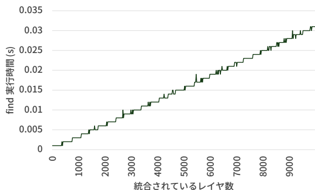
図 5: 統合されているレイヤ数とディレクトリ読み込み時間
