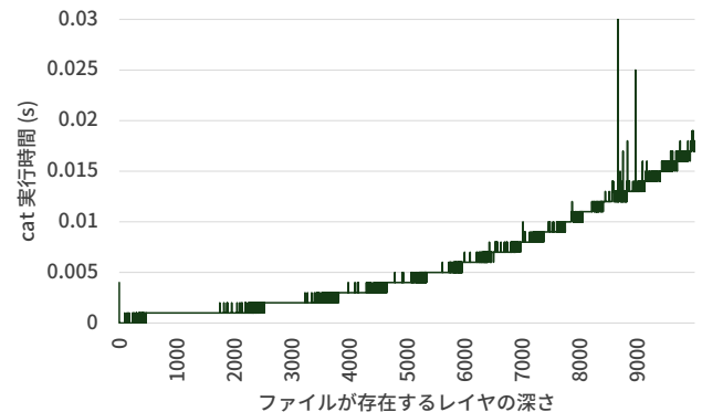
図 4: ファイルが存在するレイヤの深さと読み込み時間
