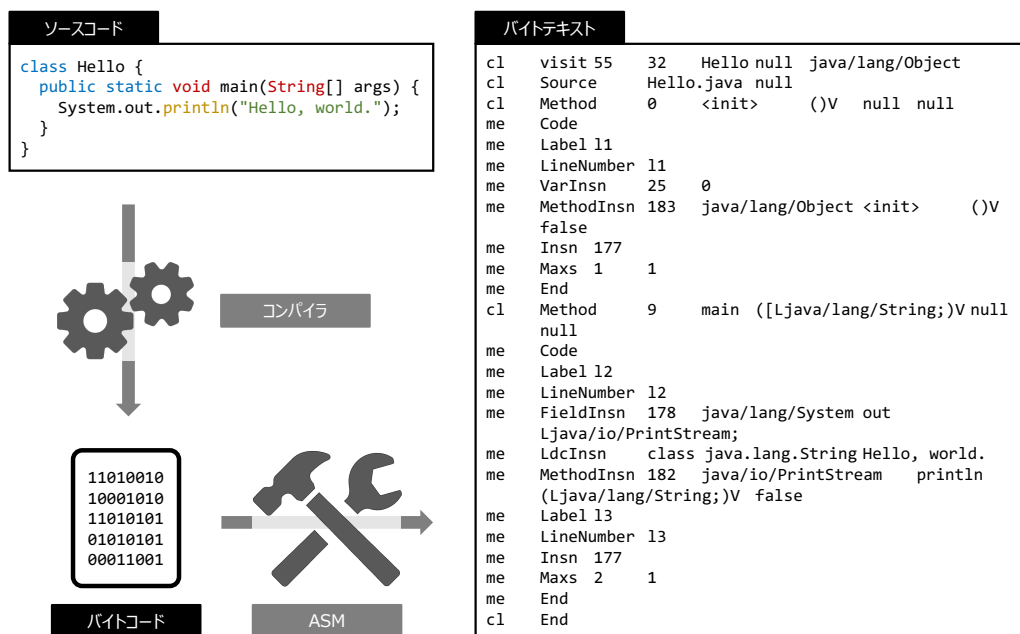
図4 ASM を利用したバイトコードからのバイトテキストの書き出し
