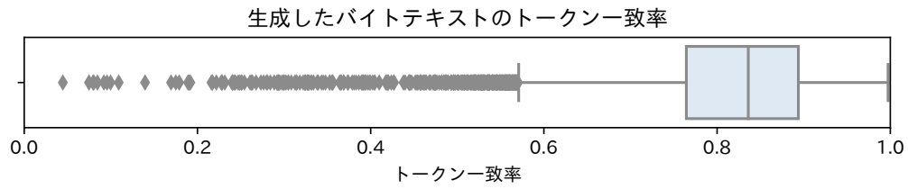
図 10 生成したバイトテキストのトークン一致率
