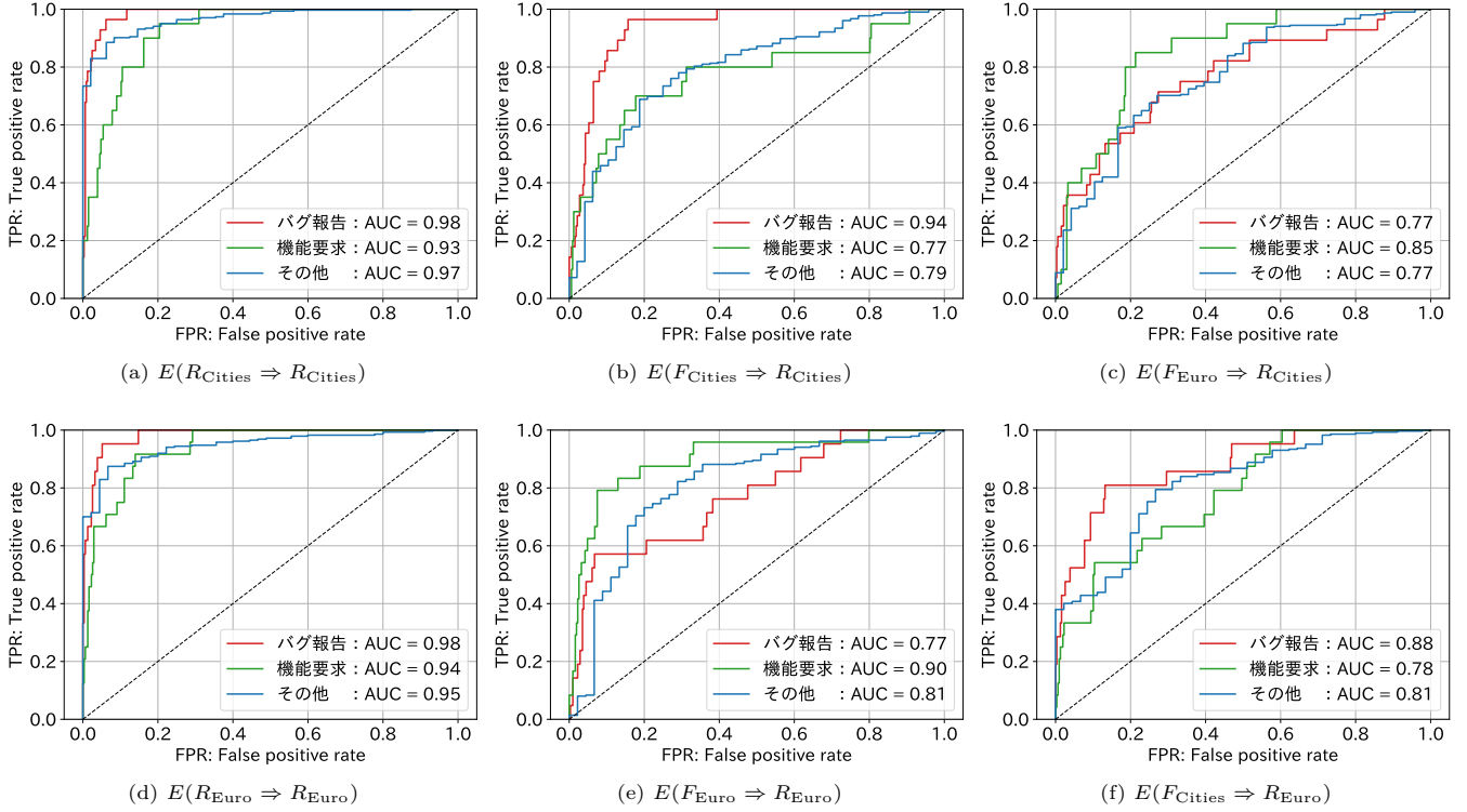
図 3 ROC 曲線
