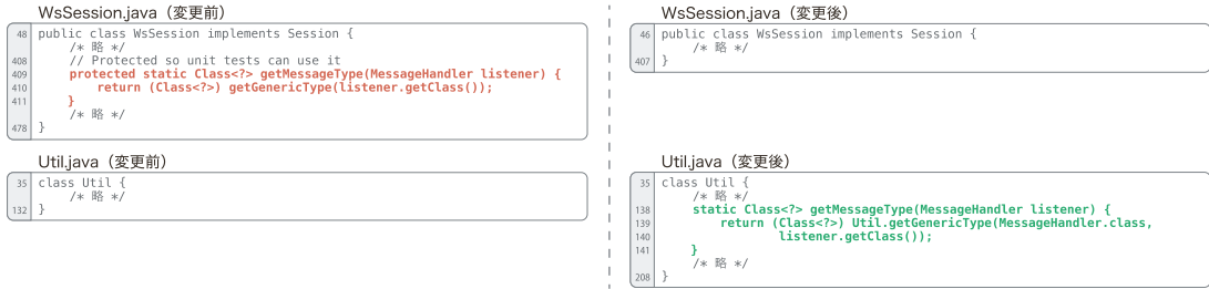
図 10 既存手法によるリファクタリング時の差分検出結果
