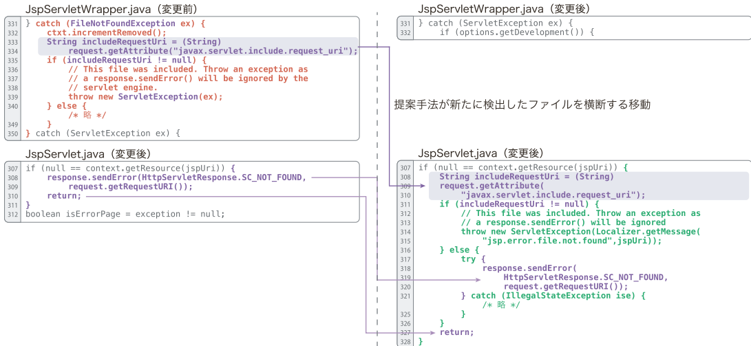
図 13 提案手法によるバグ修正時の差分検出結果
