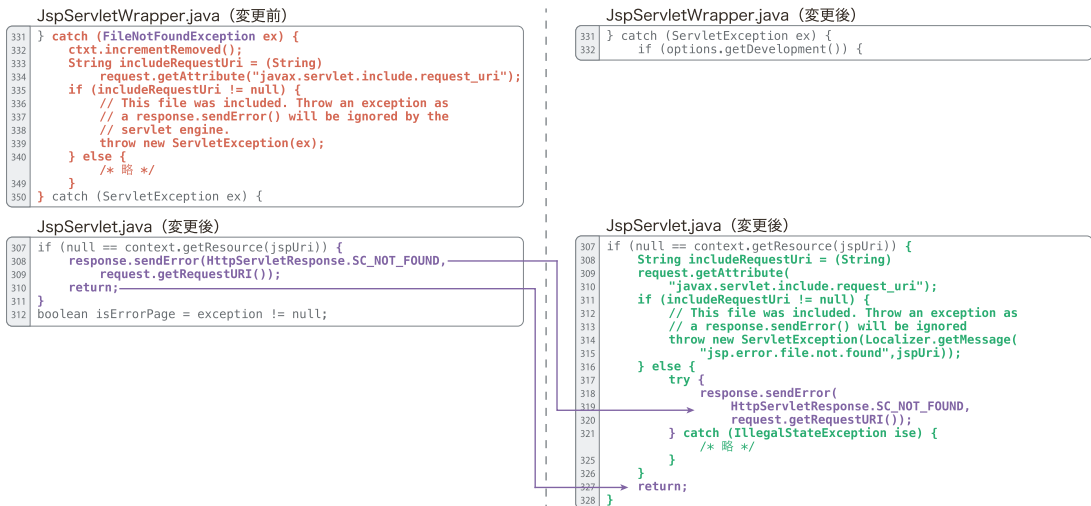
図 12 既存手法によるバグ修正時の差分検出結果
