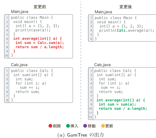
(a) GumTree の出力
