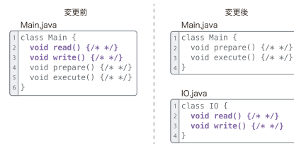
(a) 機能の分割のソースコードの例
