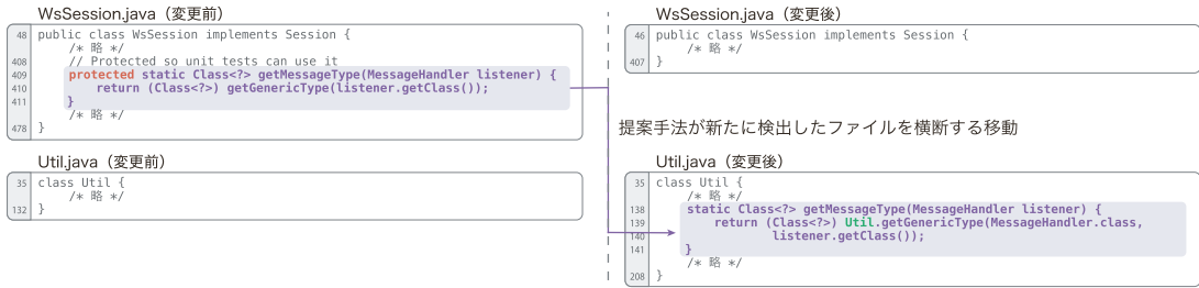
図 11 提案手法によるリファクタリング時の差分検出結果
