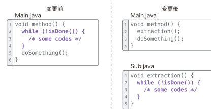
(b) メソッドへの切り出しのソースコードの例
