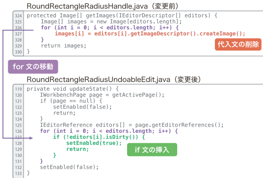
図8 移動元と移動先のソースコードが大きく異なる例
