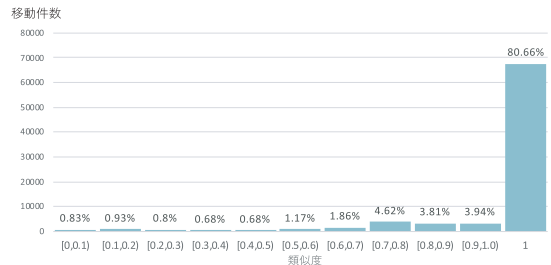
図9 移動前後のソースコード片の類似度の分布
