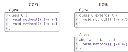
(c) 継承関係の変化のソースコードの例
