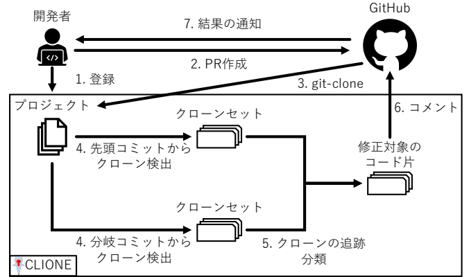
図 3: CLIONE の概要
