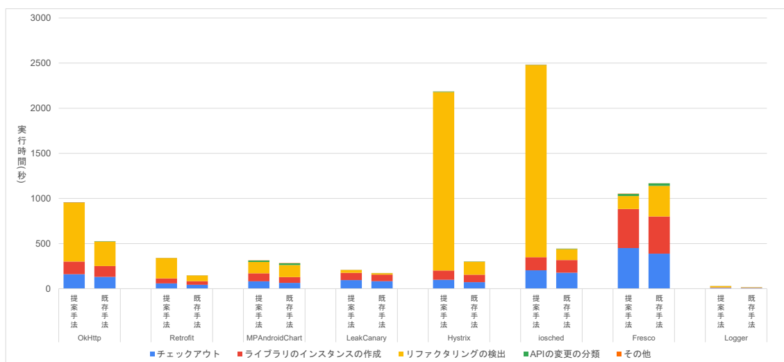
図 5 API に対する変更の検出に要する時間
