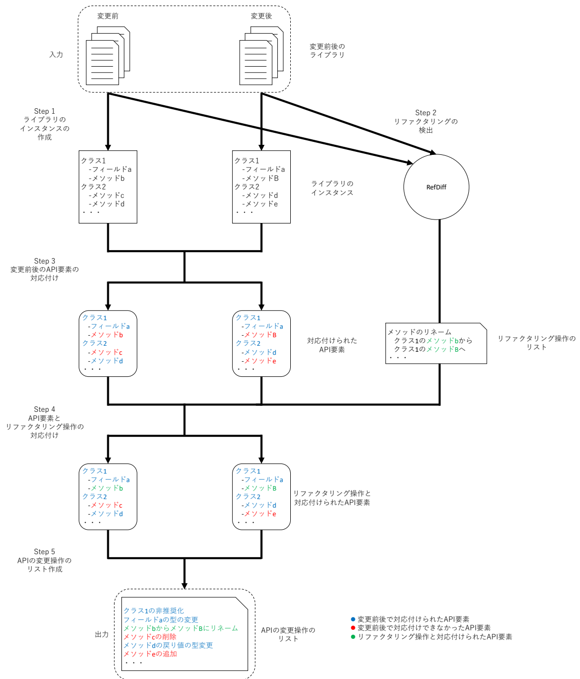
図2 APIDiffの概要
