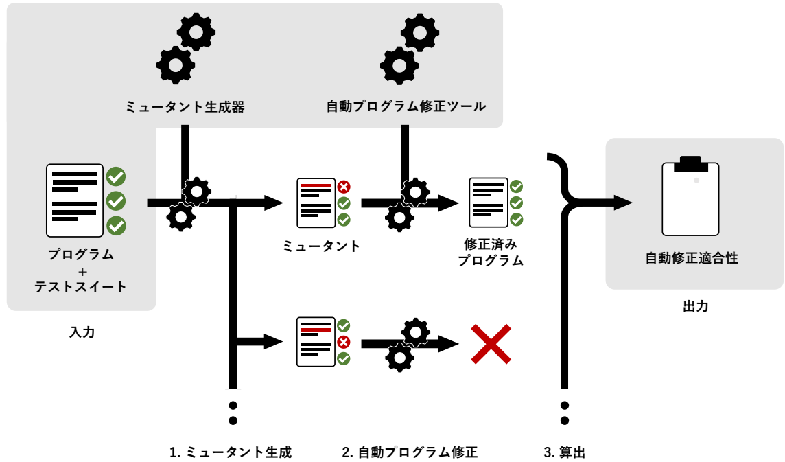
図 4 提案手法の流れ
