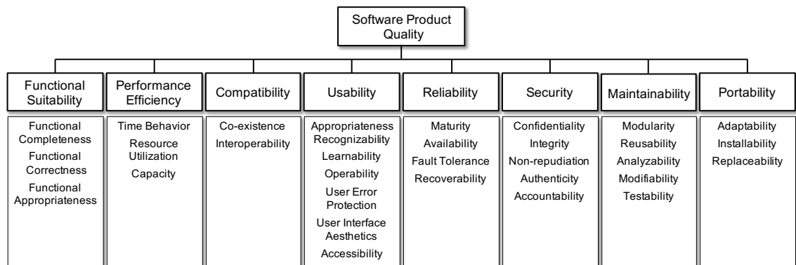
図1 ISO/IEC 25010 のソフトウェア品質モデル
