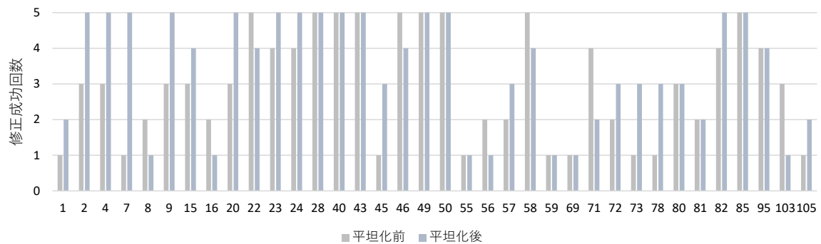
図 16 修正に成功した欠陥の修正成功回数
