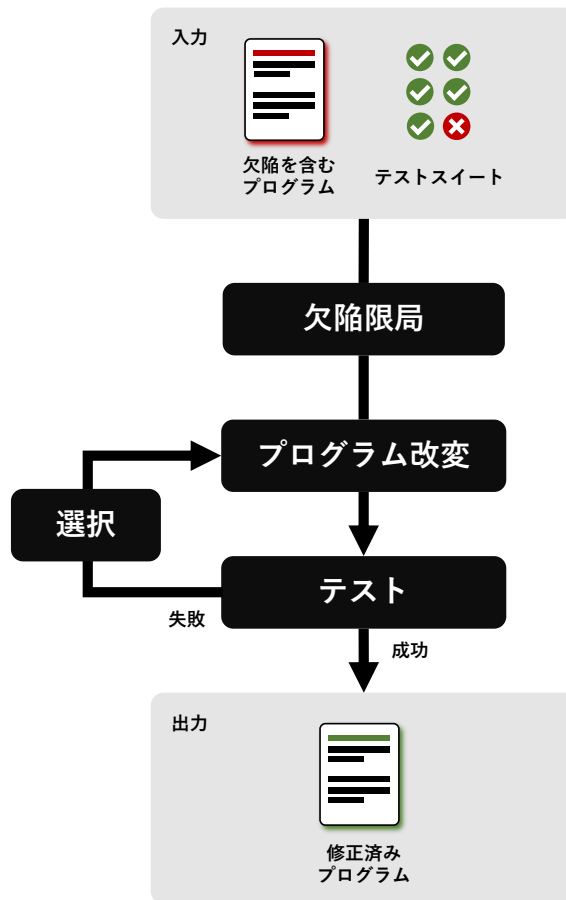
図 2 GenProg の処理の流れ
