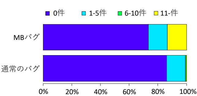
図 3 RQ1a: 重複報告件数
