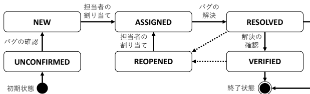
図2 BMOのバグライフサイクル
