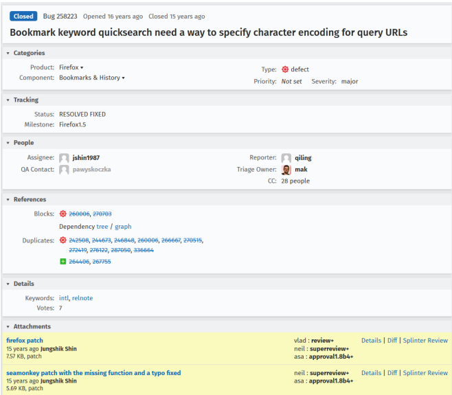
図 1 BMO のスクリーンショット
