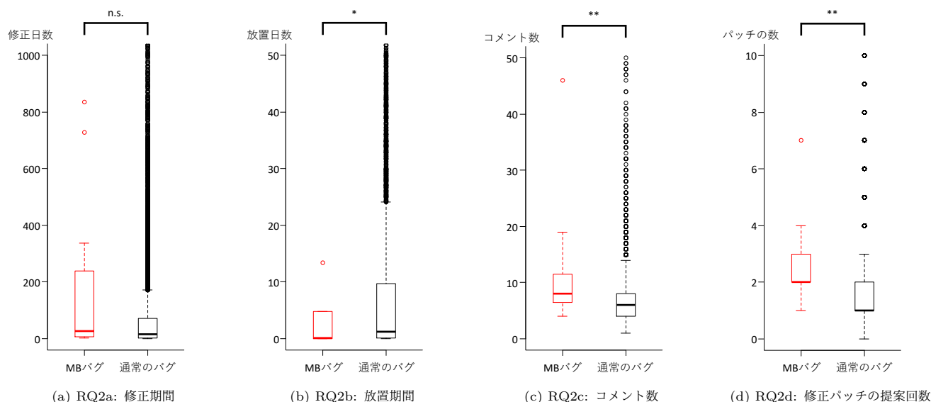
図5 RQ2の結果 (注4)
