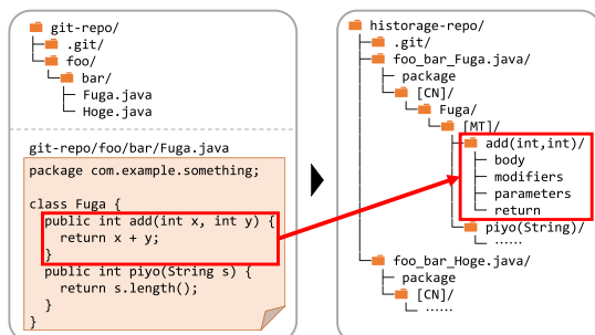
図 4 Git リポジトリ (左) を変換した Hstorage リポジトリ (右)
