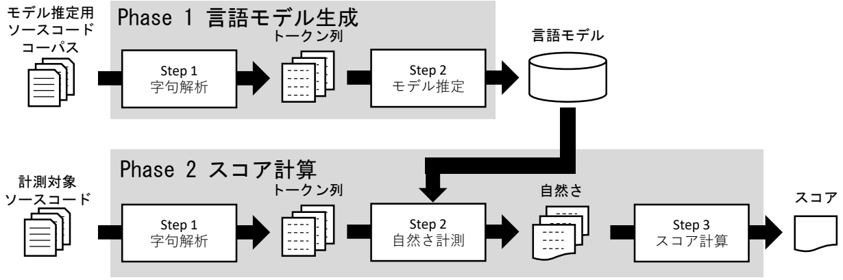
図 1 提案手法の概要
