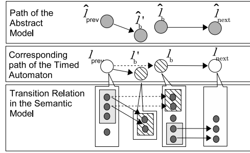
図4 洗練後のモデル
