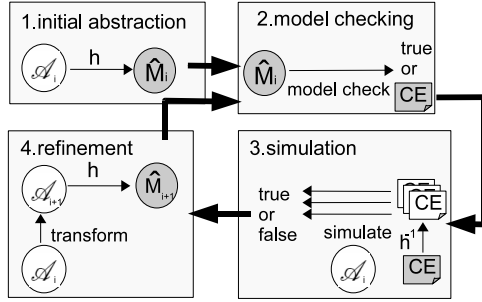
図2 これまでに提案している抽象化
