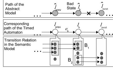
図3 反例
