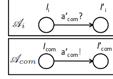
図 5 独立な遷移の同期
