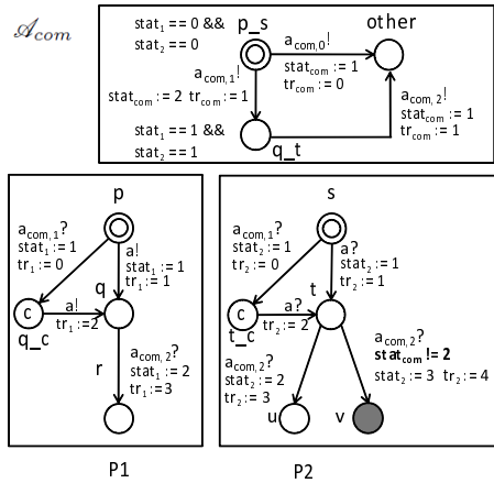
図 12 洗練後のモデル
