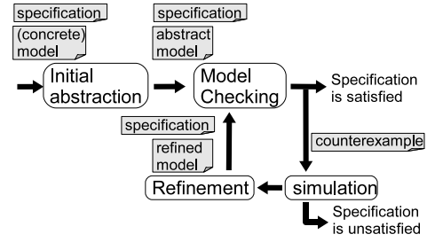
図 1 CEGAR ループ
