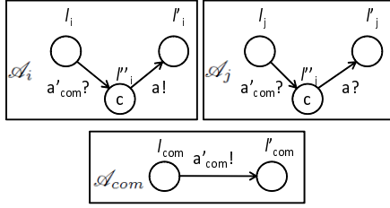
図 6 互いに同期する遷移との同期
