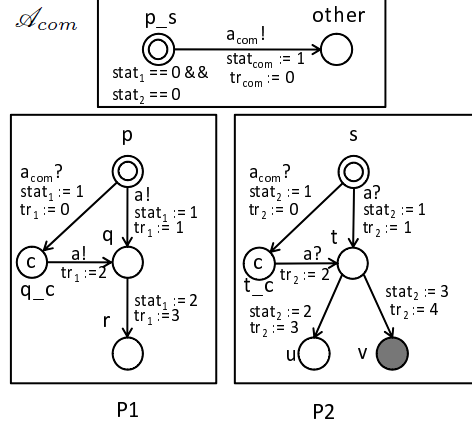
図 11 部分合成モデルを追加したモデル
