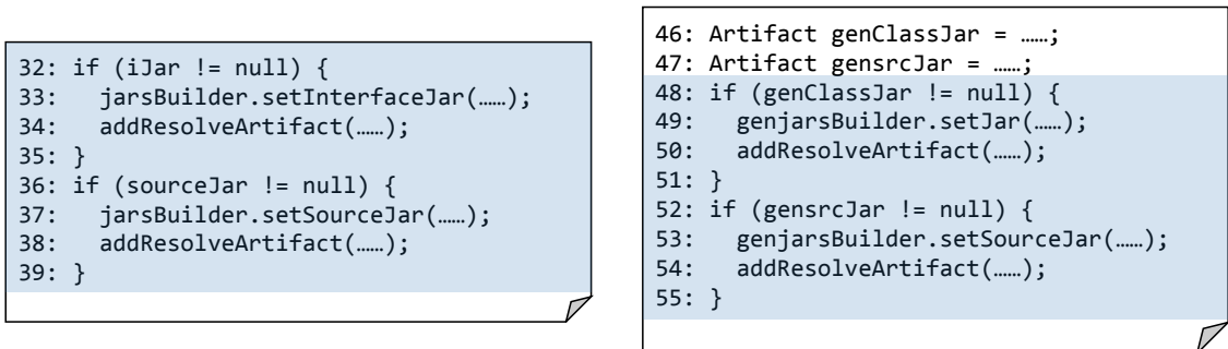
文の順序統一後のコード片
