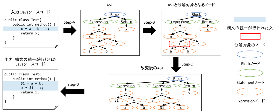
図 11: 構文の統一の例
