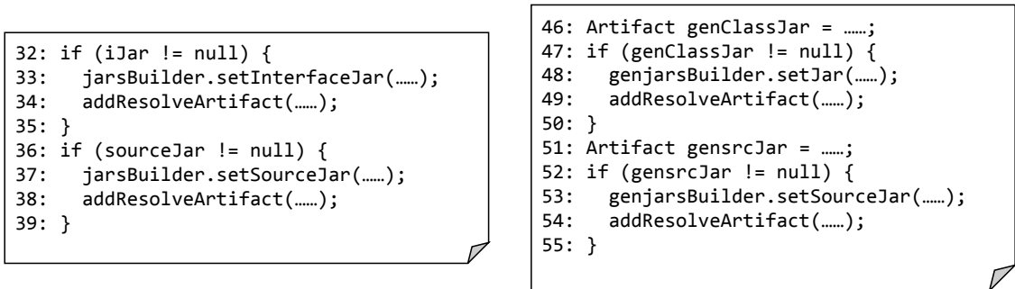
文の順序統一前のコード片
