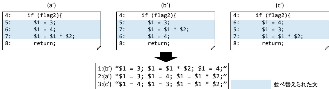
図 10: 変数名の正規化とアルファベット順のソート
