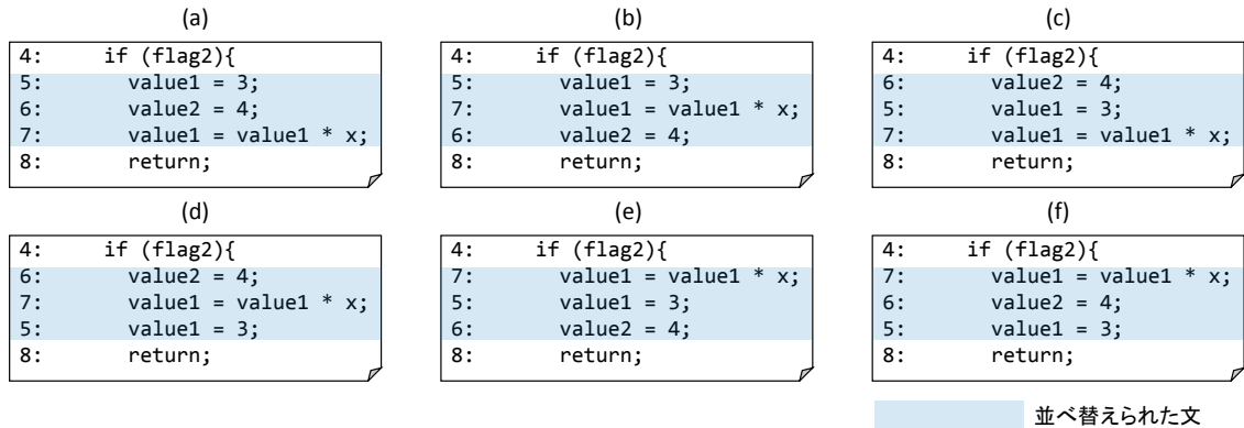
図 9: ノードの順序をそれぞれソースコードで表したもの
