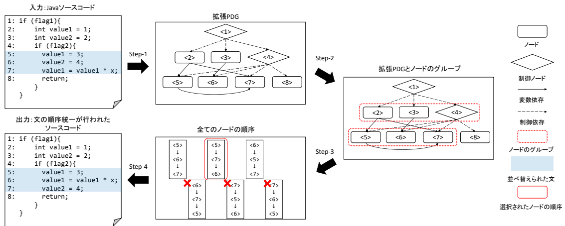
図 8: 文の順序統一の例
