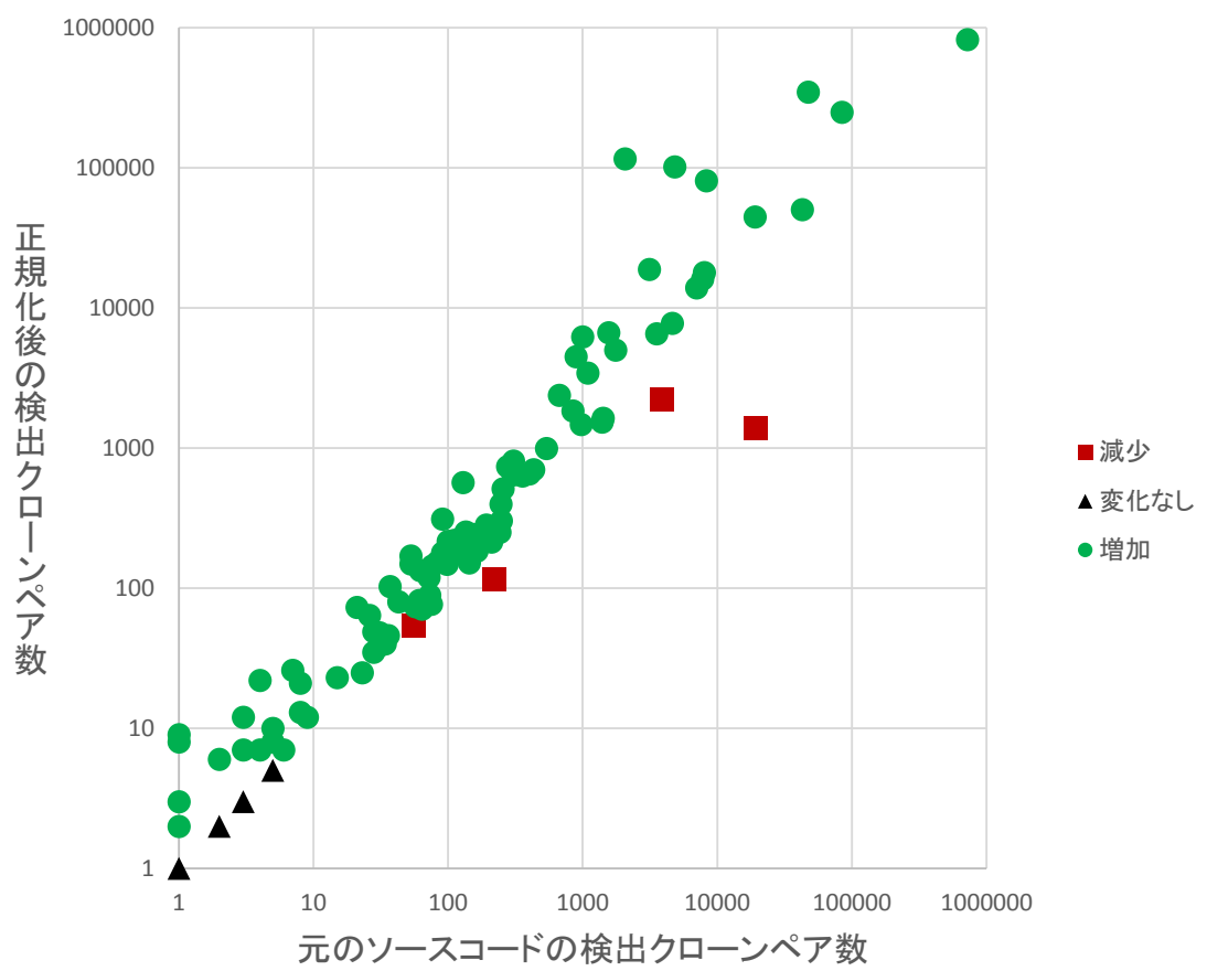
図 17: 追加実験の実験結果
