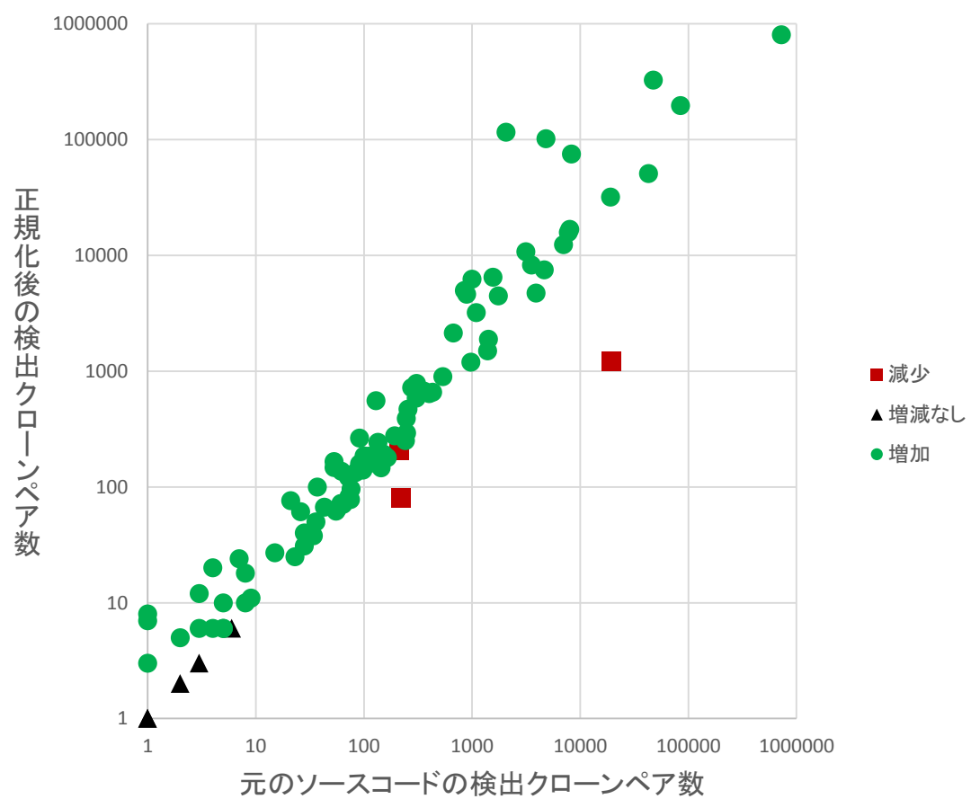
図 14: 構文の統一の実験結果
