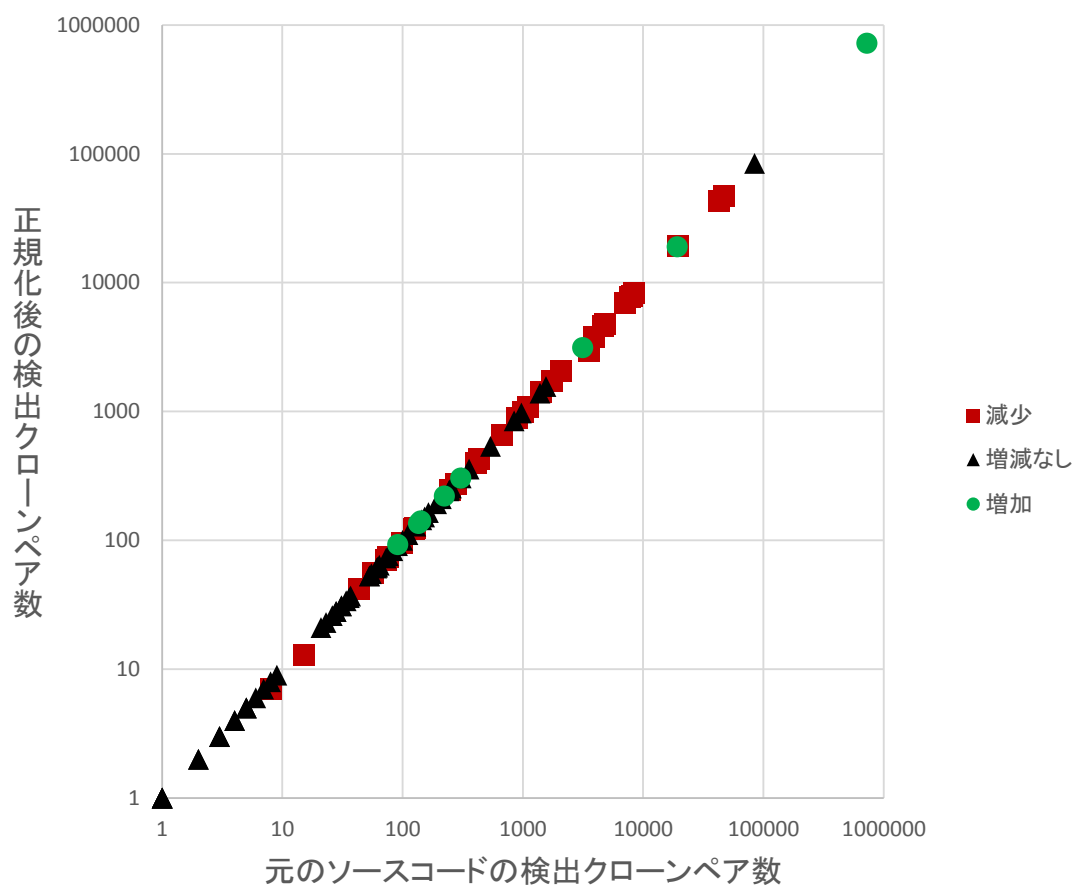
図 12: 文の順序統一の実験結果
