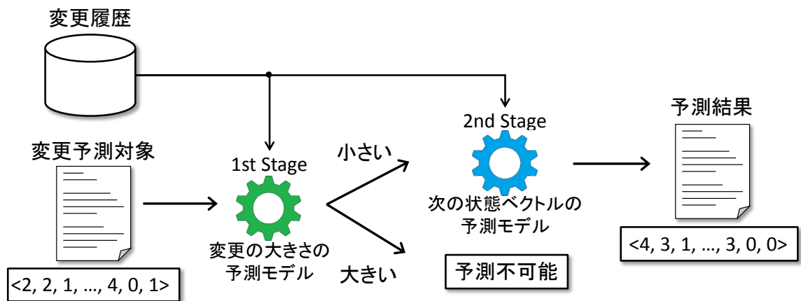
図 5: ソースコードの変更予測手法の概要
