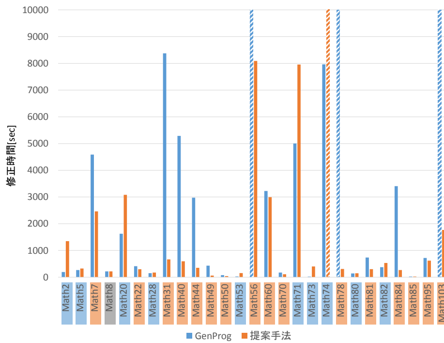
図 9: 実験結果 (seed=0)
