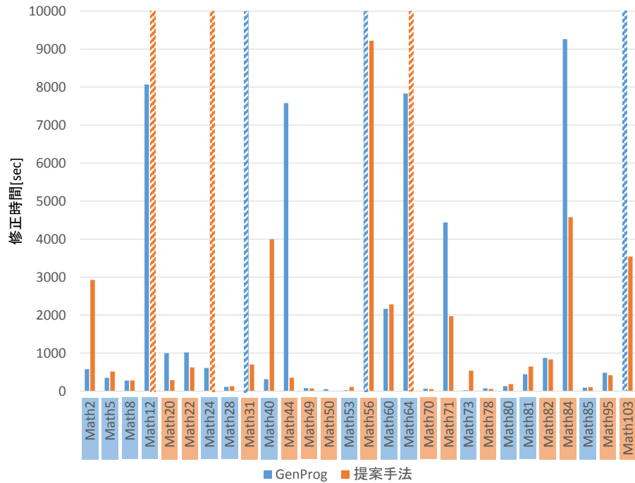
図 11: 実験結果 (seed=2)
