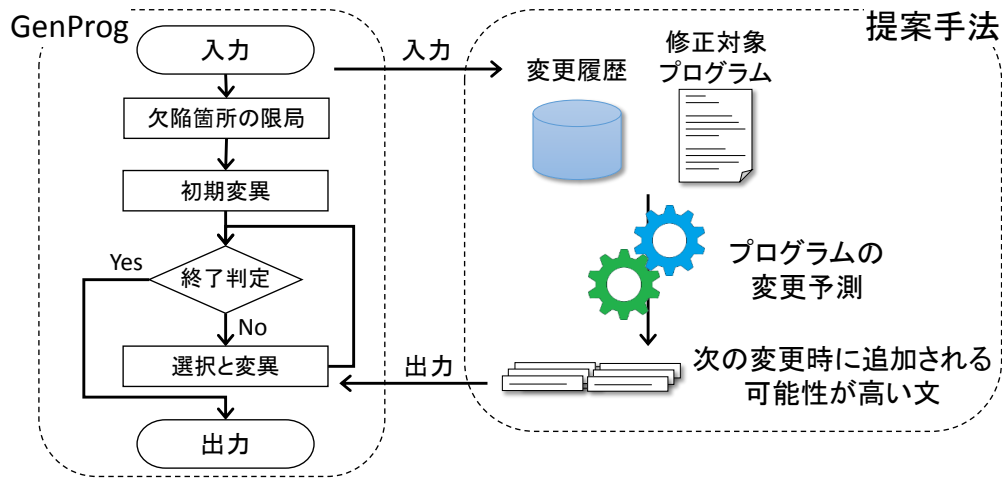
図 6: 提案手法の概要
