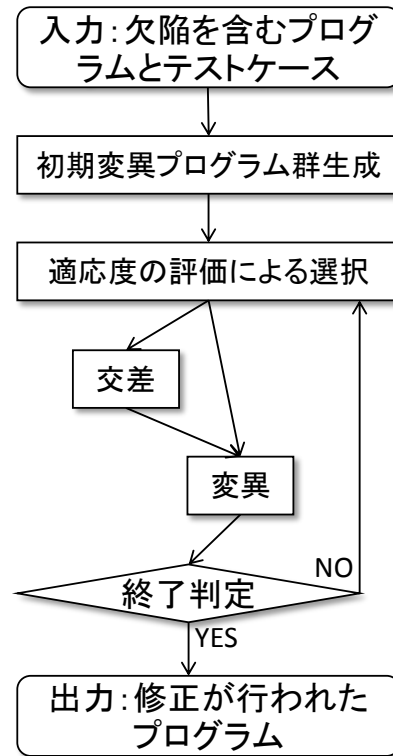
図 3: GenProg の動作の流れ
