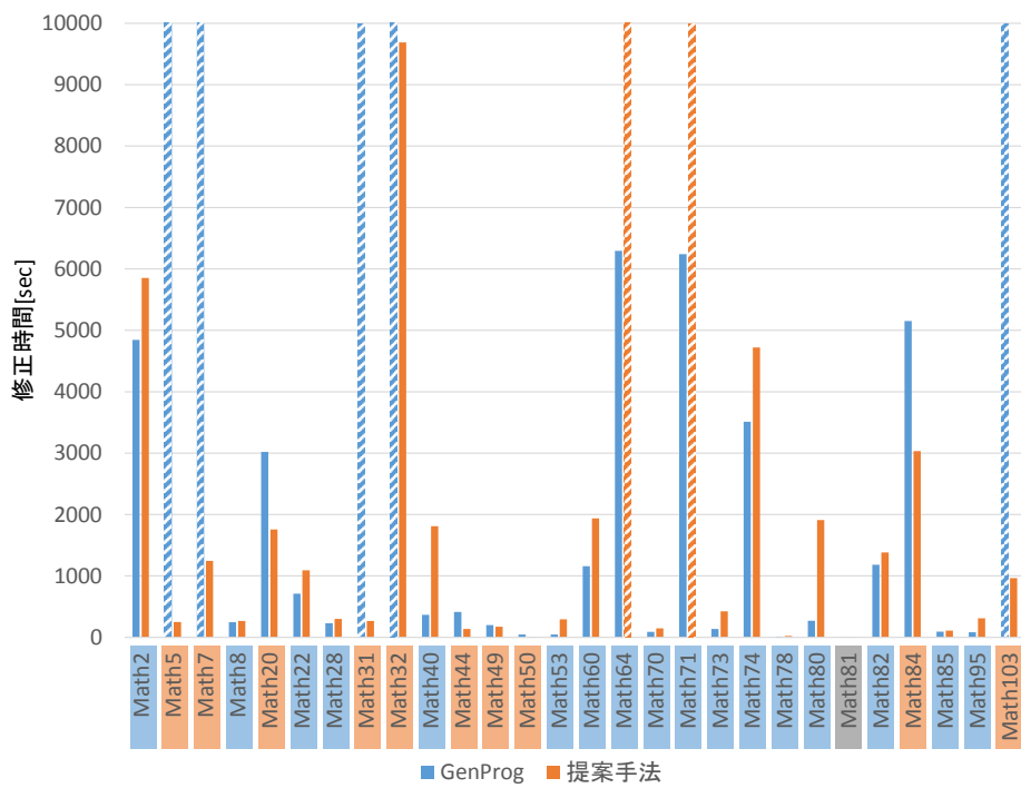
図 10: 実験結果 (seed=1)
