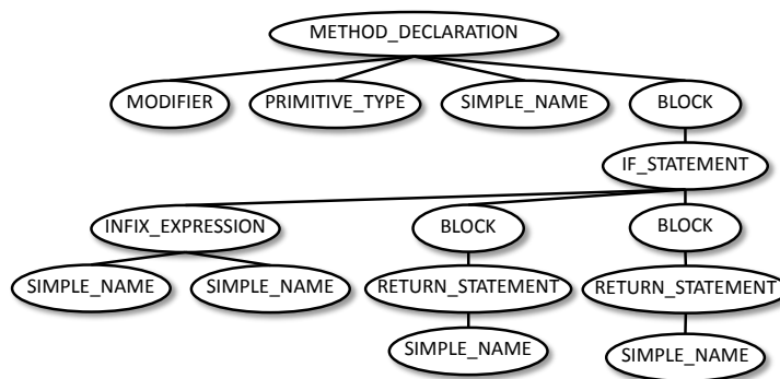
(b) 抽象構文木
