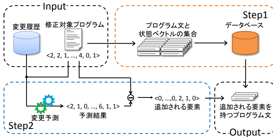
図 7: 提案手法の詳細
