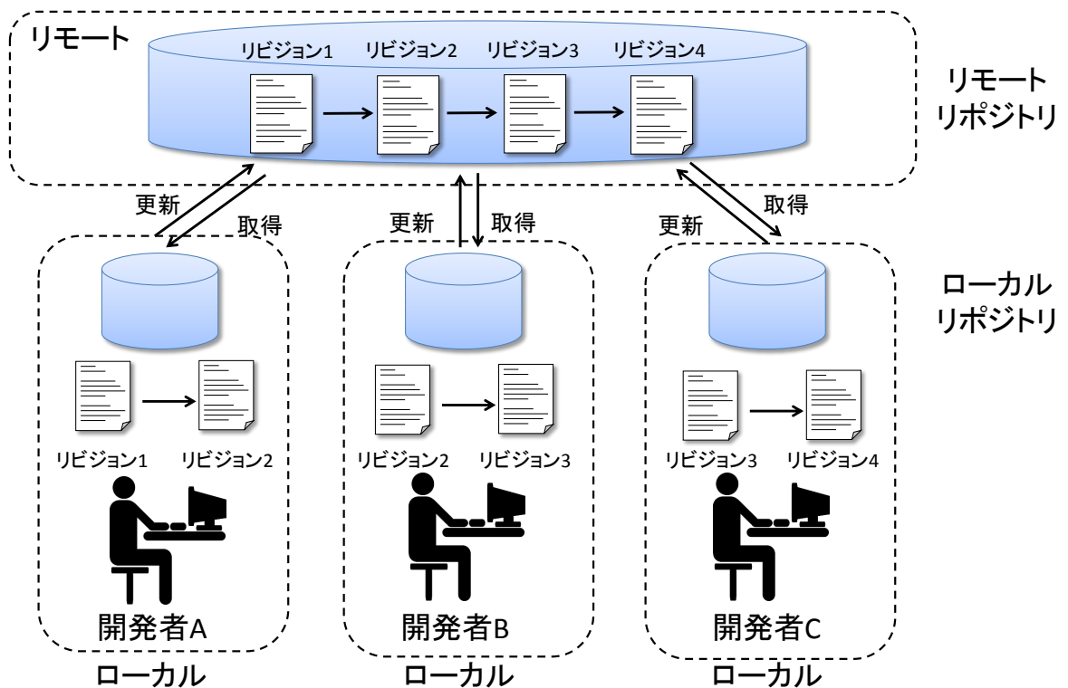
図 1: バージョン管理システム
