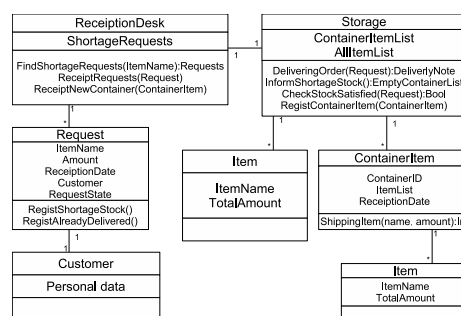
図 1 在庫管理プログラムのクラス構成
