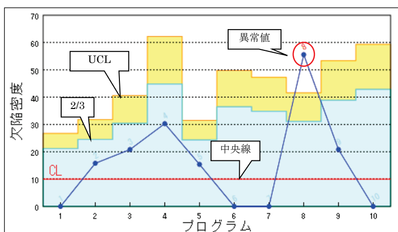
図 8. 検出欠陥密度の u 管理図
