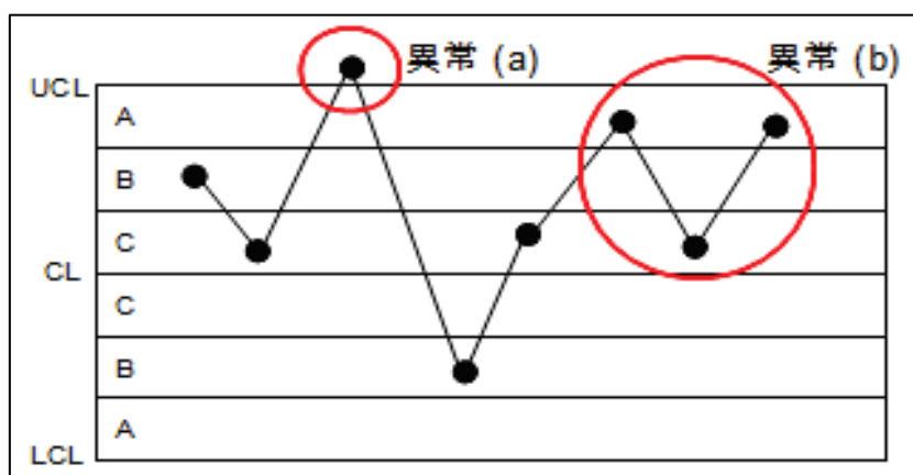
図 7. X 管理図のサンプル
