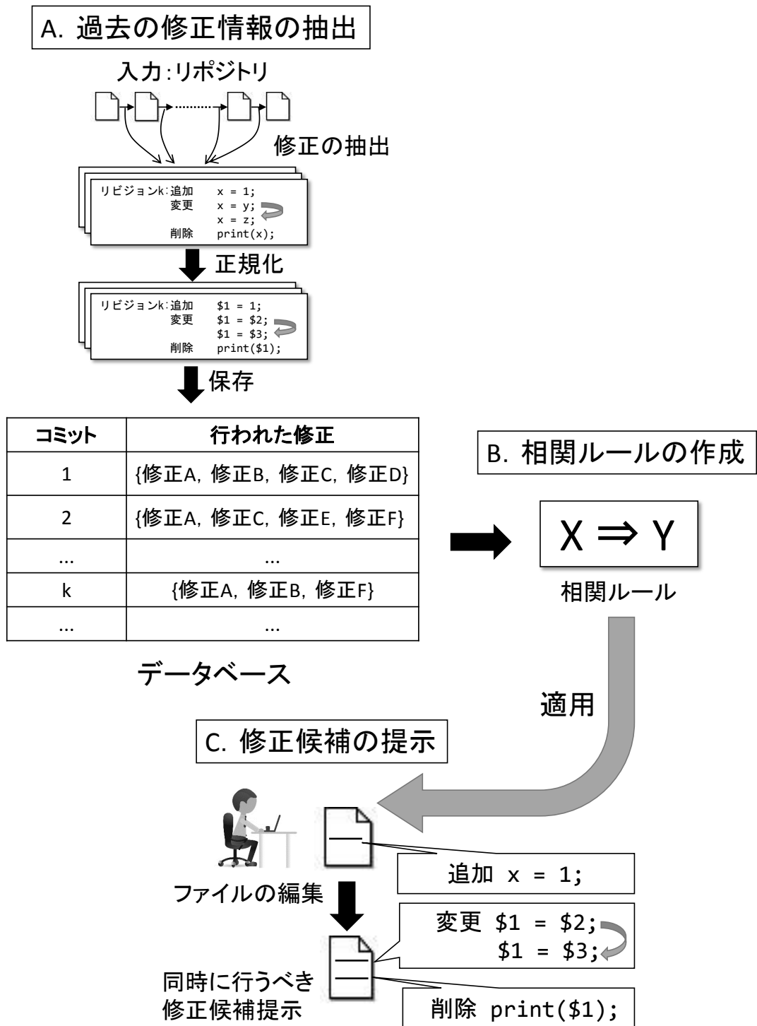
図 2: 提案手法の概要
