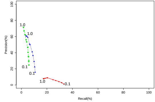
(d) ArgoUML
