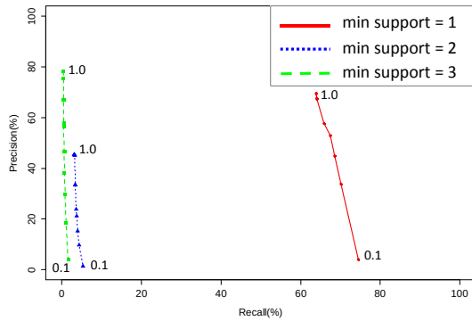
(a) FreeBSD
