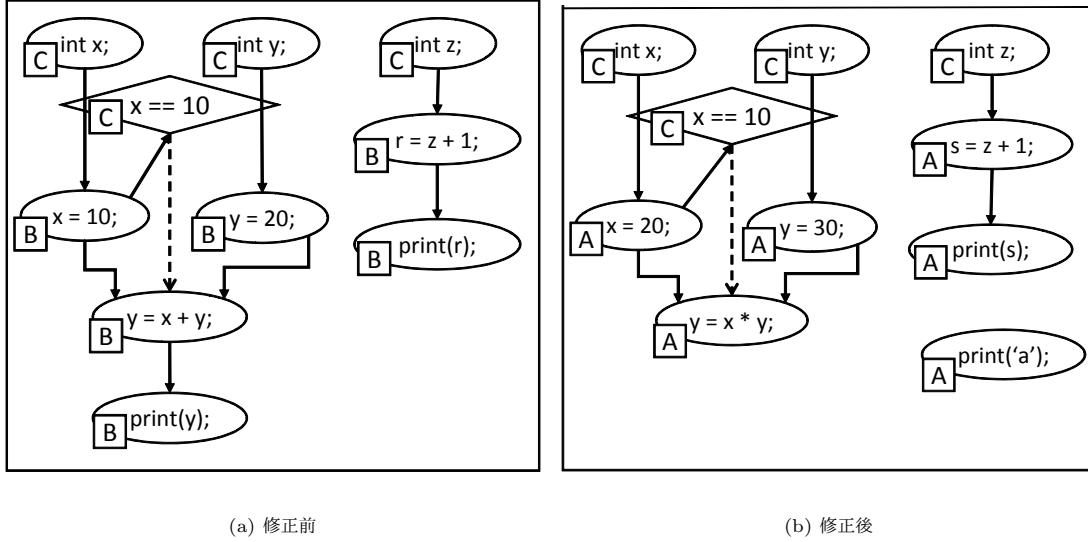
図 2 修正前後の PDG
