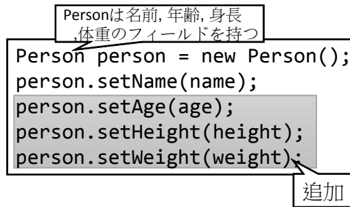
図 8 修正が不適切に分割されてしまう例
