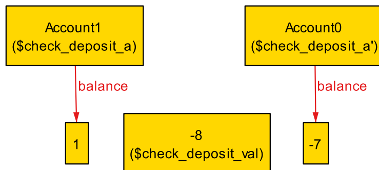
図 4: Alloy Analyzer の解析結果の例 ( check_deposit )
