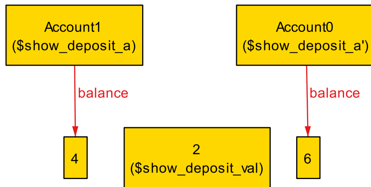
図 3: Alloy Analyzer の解析結果の例 ( show_deposit )
