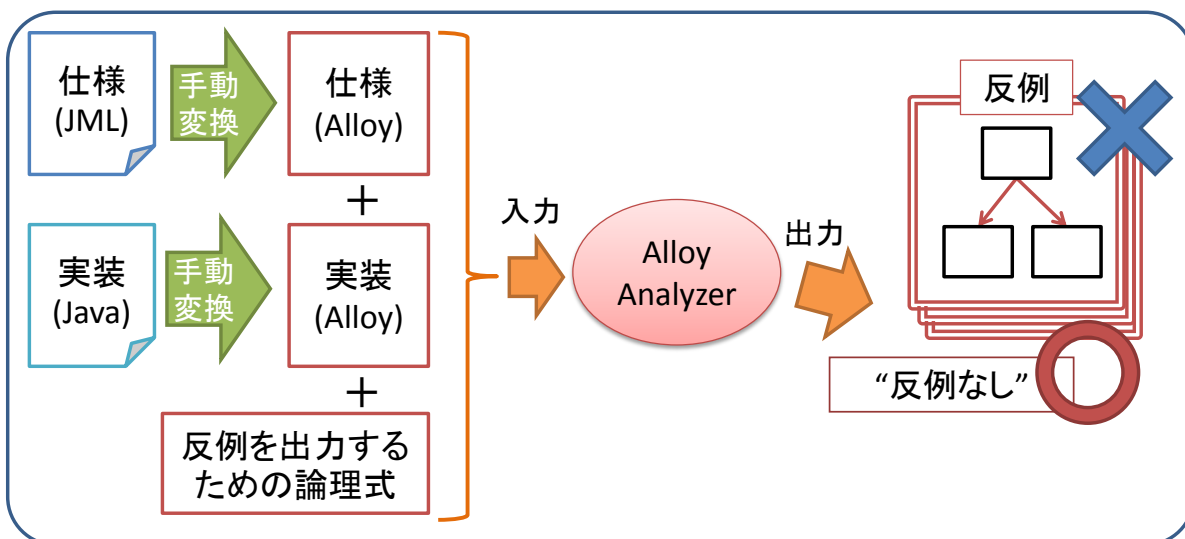
(b) 実装と表明との不一致の検出
