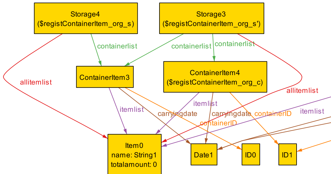
図 18: 反例 (registContainerItem()(updateAllItemList()))
