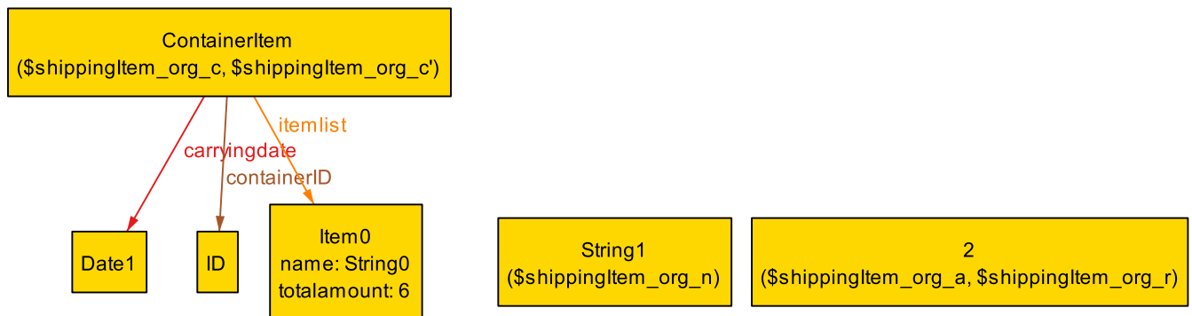
図 17: 反例 (shippingItem())
