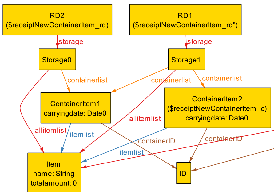
图 20: 反例 (receiptNewContainerItem())
