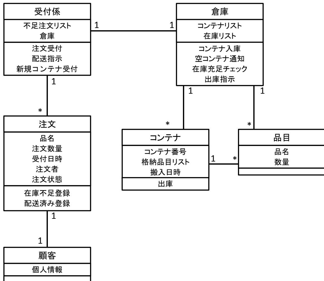
図 14: 対象プログラムのクラス図
