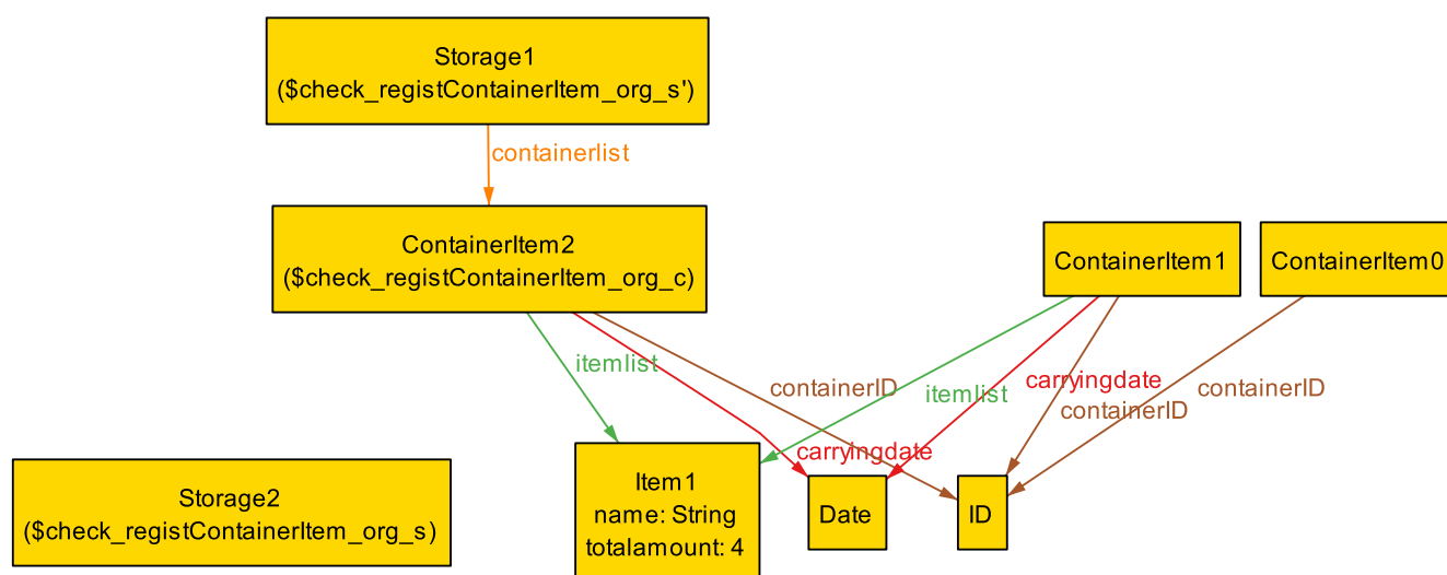
図 16: 充足例 (registContainerItem())
