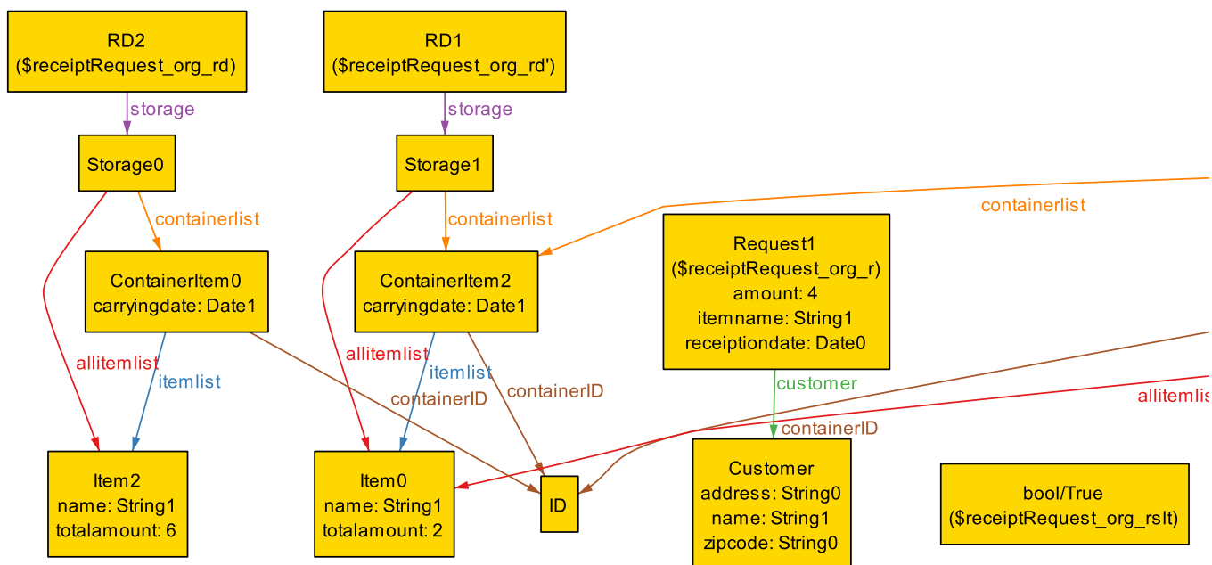
图 19: 反例 (receiptRequest())
