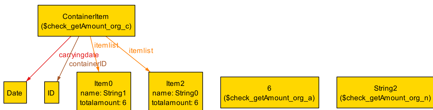
図 15: 充足例 (getAmount())
