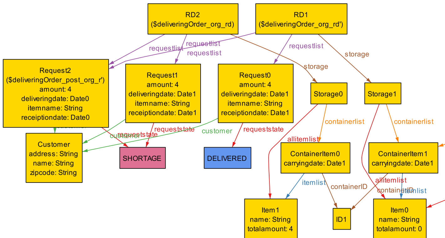
図 21: 反例 (deliveringOrder())
