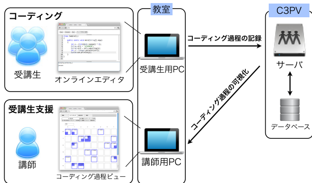
図 1 コーディング過程可視化システム C3PV の概要
