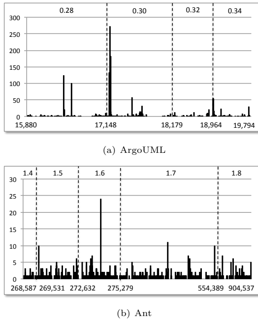
図 4 コードクローンの消失数
