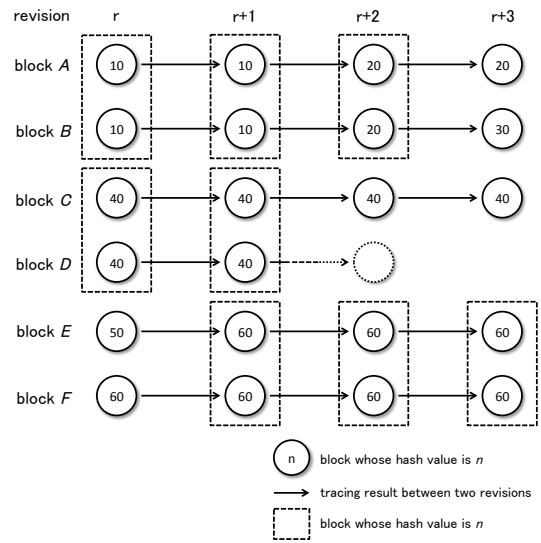
図 3 コードクローンの消失の特定例
