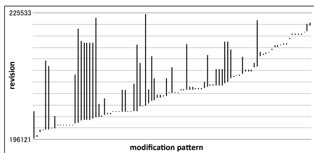
(b) FreeBSD
