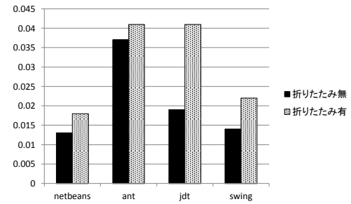
(b) okprecision
