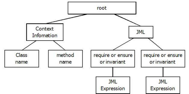
図 8 コンテキスト宣言を含む JML 抽象構文木
